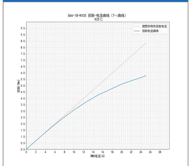
G66-18-KV35 扭矩 - 电流曲线 (T-i 曲线) @25°C
