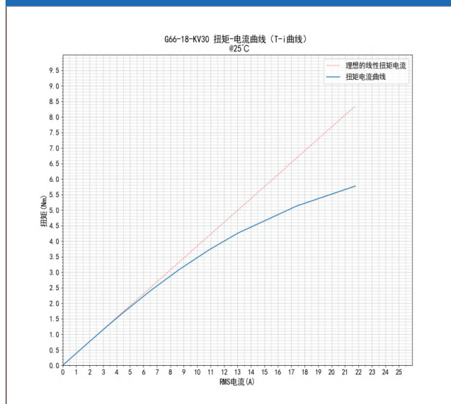
G66-18-KV30 扭矩 - 电流曲线 (T-i 曲线) @25°C
