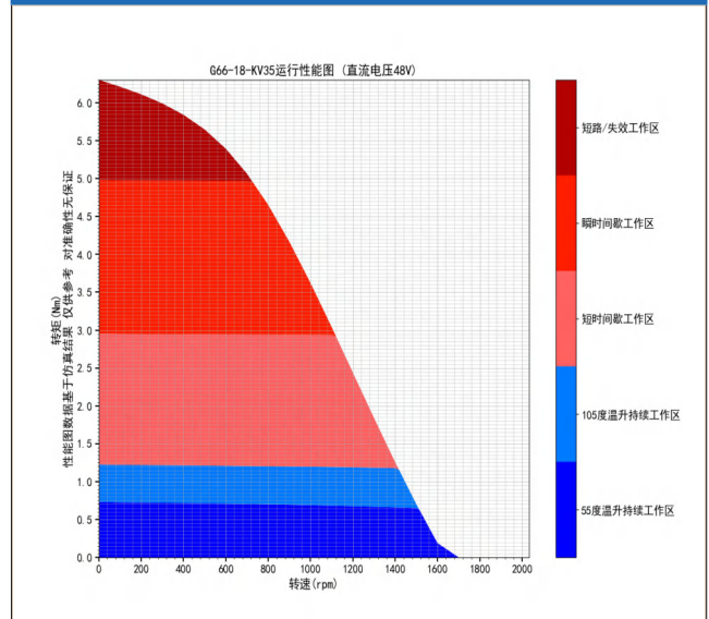
G66-18-KV35 运行性能图 (直流电压48V)
