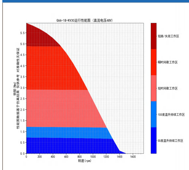
G66-18-KV30 运行性能图 (直流电压48V)
