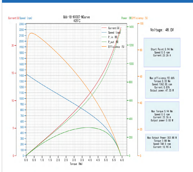
G66-18-KV30 T-NCurve@25C
