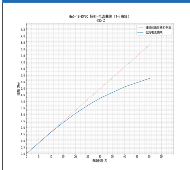
G66-18-KV70 扭矩 - 电流曲线 (T-i 曲线) @25°C
