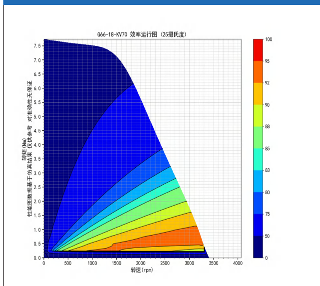
G66-18-KV70 效率运行图 (25摄氏度)
