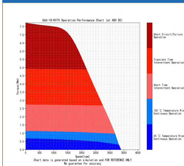
G66-18-KV70 运行性能图 (直流电压48V)
