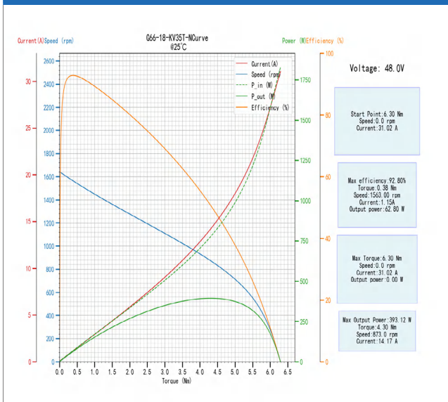
G66-18-KV35 T-NCurve@25C
