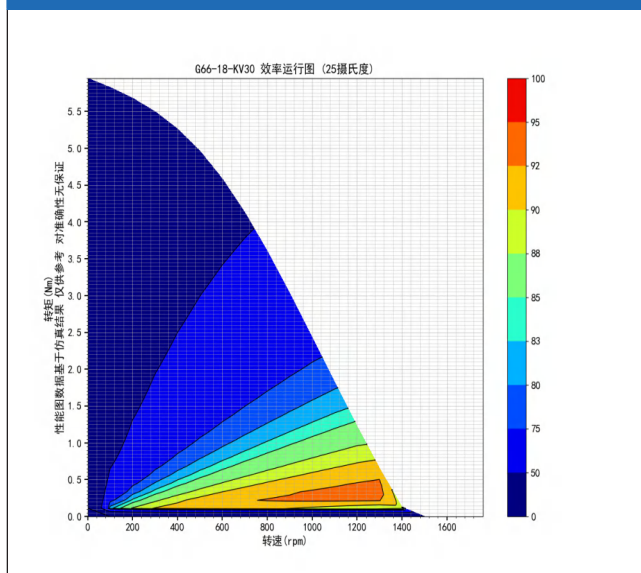
G66-18-KV30 效率运行图 (25摄氏度)
