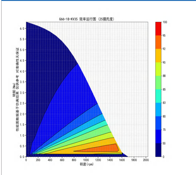
G66-18-KV35 效率运行图 (25摄氏度)
