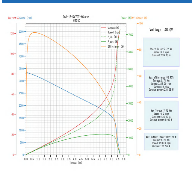
G66-18-KV70 T-NCurve@25C
